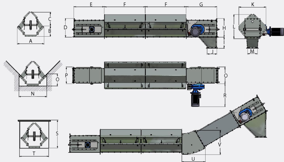
Målskitse T49/T57:
